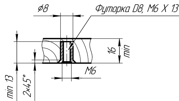
Рис. 1 Вариант отверстия в столешнице для винта М6х12 под футорку D8, М6х13. Футорка в комплект не входит!
